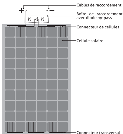
Schéma du module face avant
